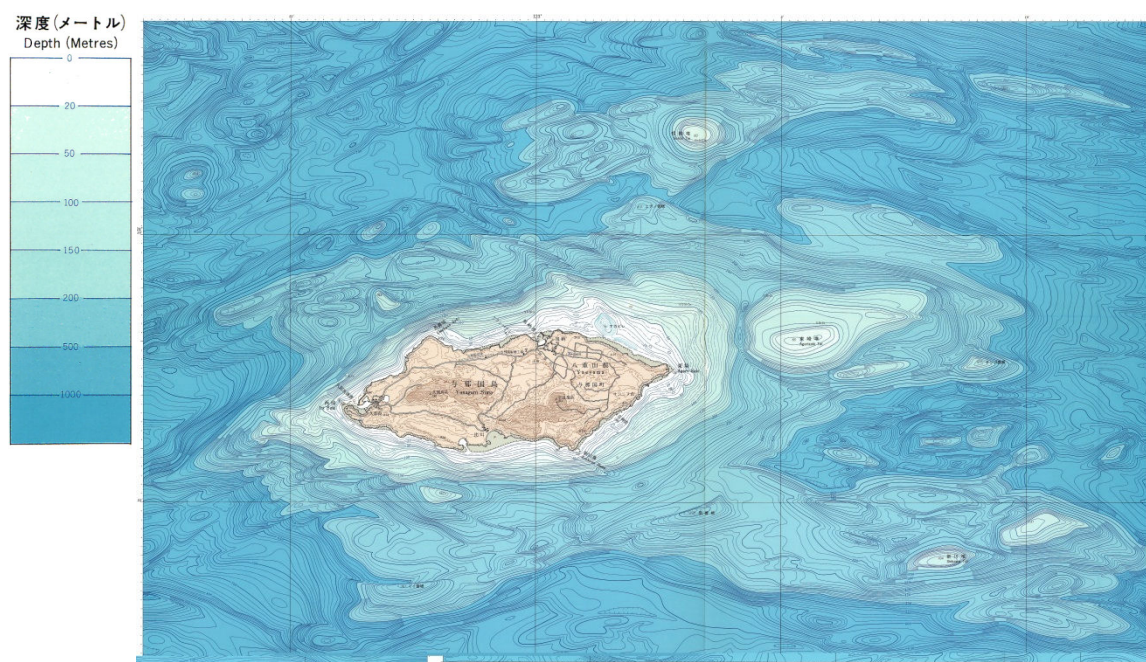
与那国島周辺の海底地形
